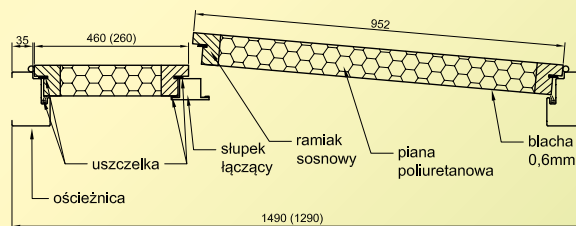
Przekrój poziomy przez drzwi dwuskrzydłowe
