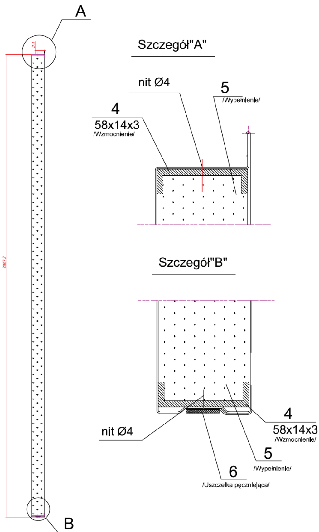
Rys. 13. Skrzydło drzwi typu DP1-P – przekrój pionowy
