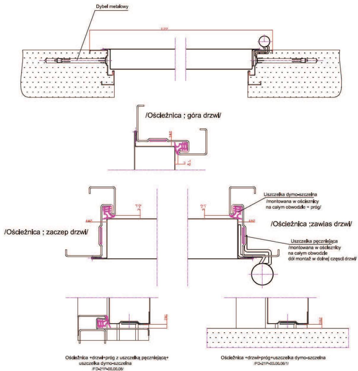
Rys. 11. Drzwi typu DP1-P przekroje i zabudowa
