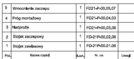
Rys. 10. Ościeżnica ze wzmocnieniem zaczepu do drzwi typu DP1-P
