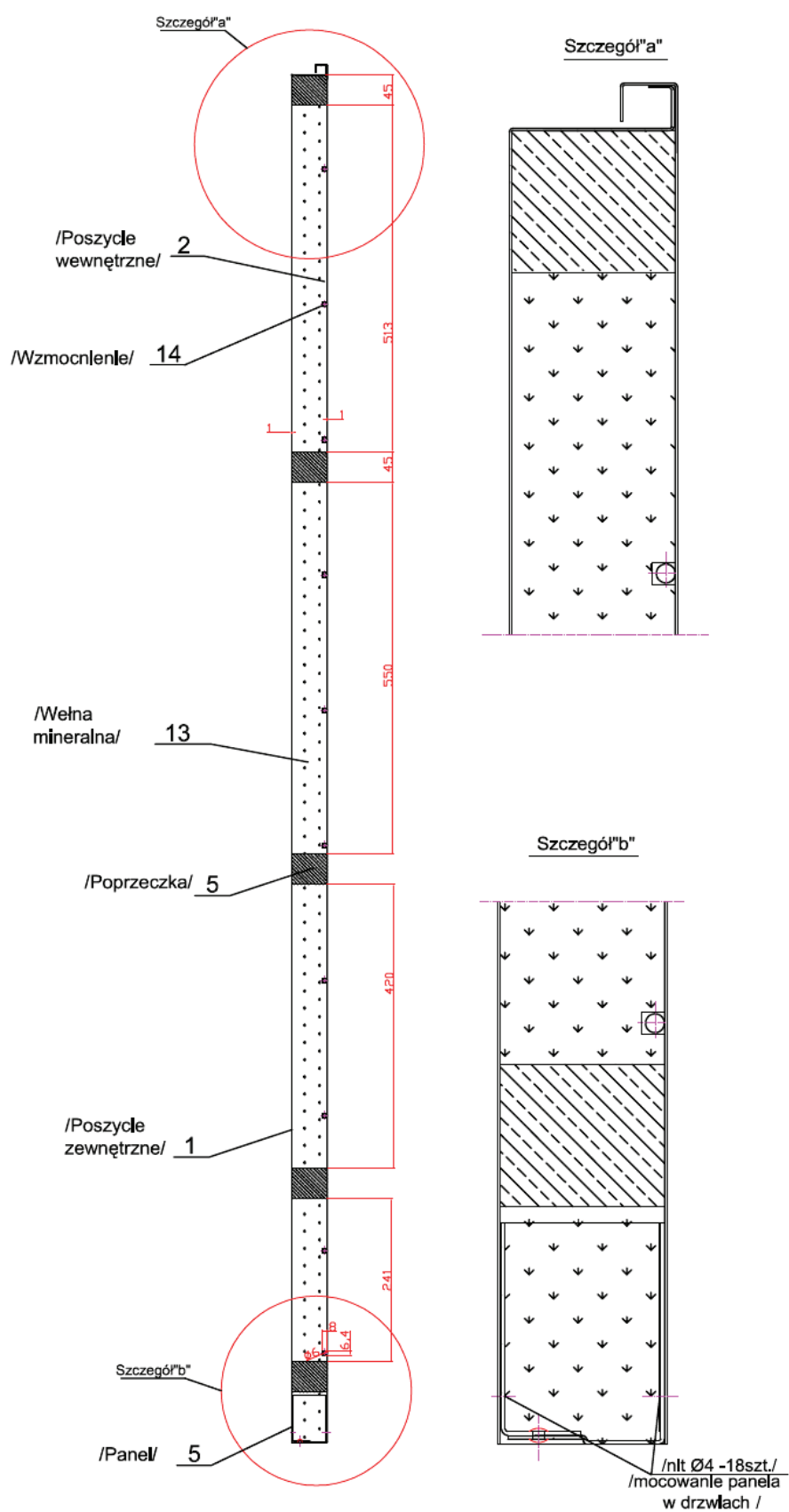
Rys. 5. Przekrój pionowy skrzydła drzwi typu SOBIESKI
