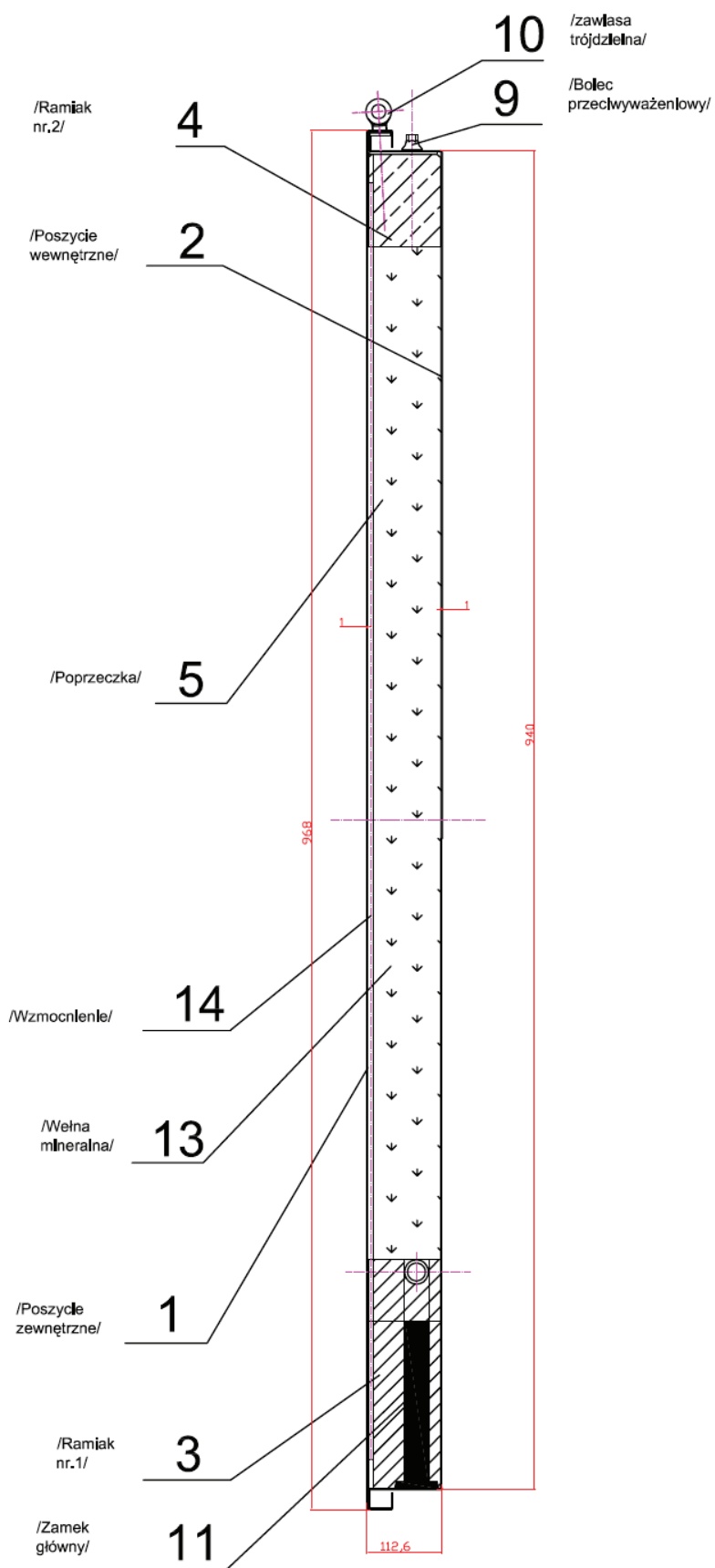
Rys. 6. Przekrój poziomy skrzydła drzwi typu SOBIESKI
