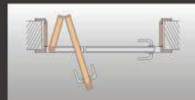
Drzwi łamane asymetryczne BEZPRZYLGOWE (lewe)
