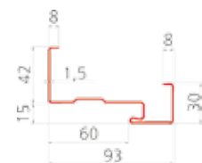
Ościeznica do drzwi przeciwpożarowych DP1-P EI30/E60
