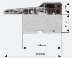
Drzwi Energooszczędne (pasywne) – grubość 100 mm – zawias widoczny
