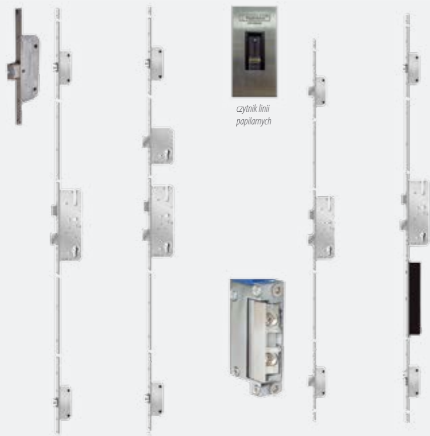
Zamek automatic 3 punktowy (standard)
