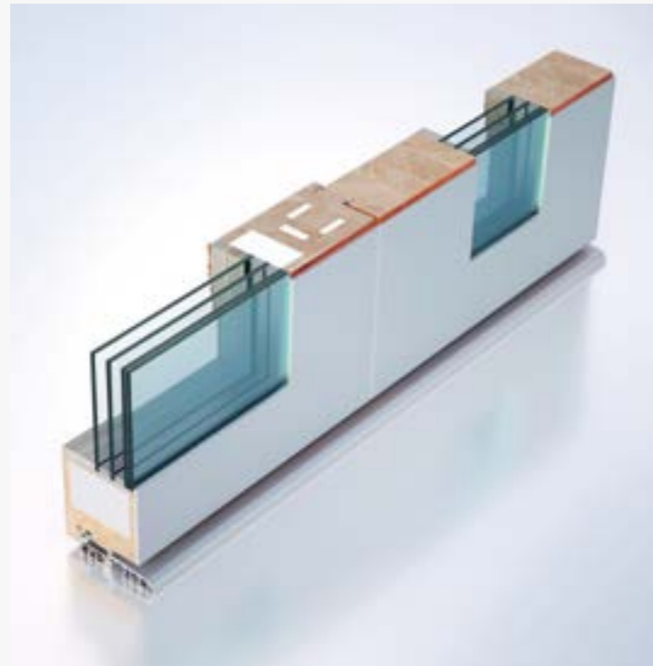
przekrój drzwi aluminiowych z dostawką, gr. 102 mm, drzwi otwierane tylko do środka, dostawka licuje się z ościeżnicą, aluminium na skrzydle, ościeżnicy i dostawce od zewnątrz
