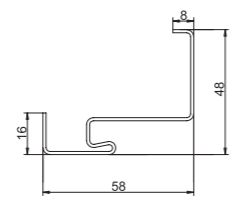
Ościeżnica BORD STALOWA narożna
