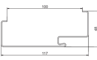
Ościeżnica BORD STALOWA stała
