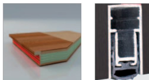
Wzmocniona ognioodporna konstrukcja skrzydeł drz. p.poż
