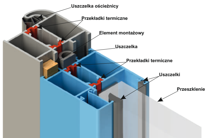
Profil ościeznicy ENERGY 60
