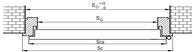
PRZEKRÓJ SKRZYDŁA - PL (gr. 42 mm)
