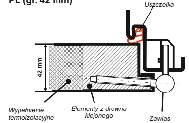
PRZEKRÓJ SKRZYDŁA - PL (gr. 42 mm)
