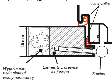
PRZEKRÓJ SKRZYDŁA - P.poż. EI 30 (gr. 46 mm)
