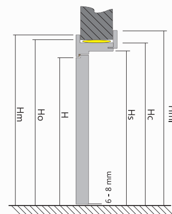
Przekrój pionowy drzwi
