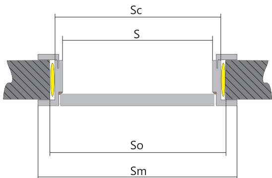
Przekrój poziomy drzwi
